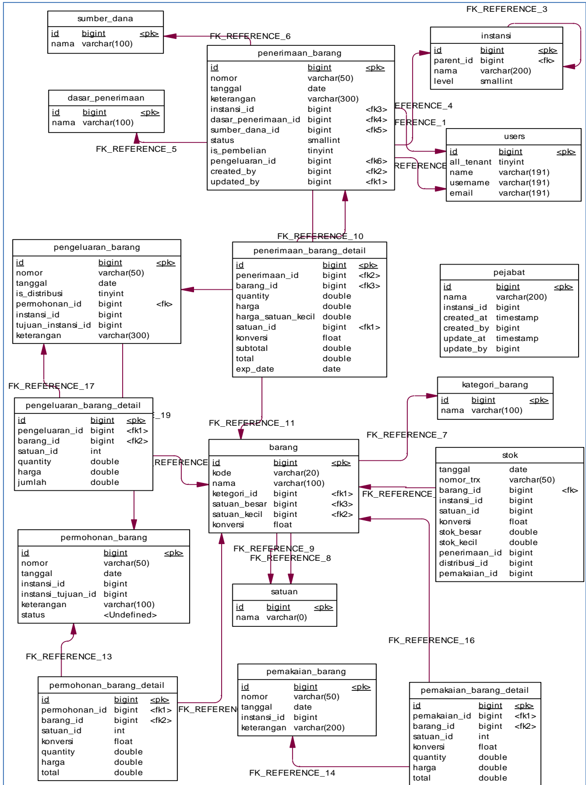
Gambar 6 Skema Database
