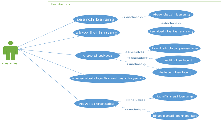
Gambar 4. Use Case Diagram Kelola Pembelian oleh Member
