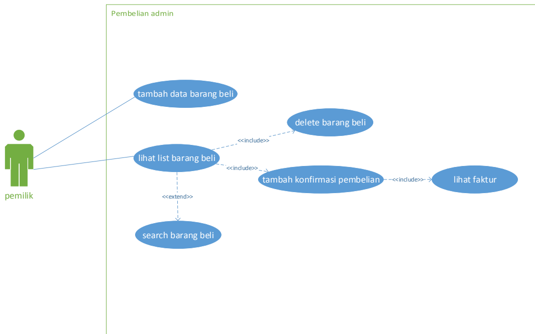
Gambar 5. Use Case Diagram Kelola Pembelian oleh Admin
