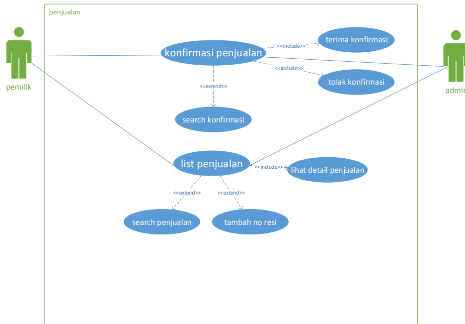
Gambar 7. Use Case Diagram Kelola Penjualan
